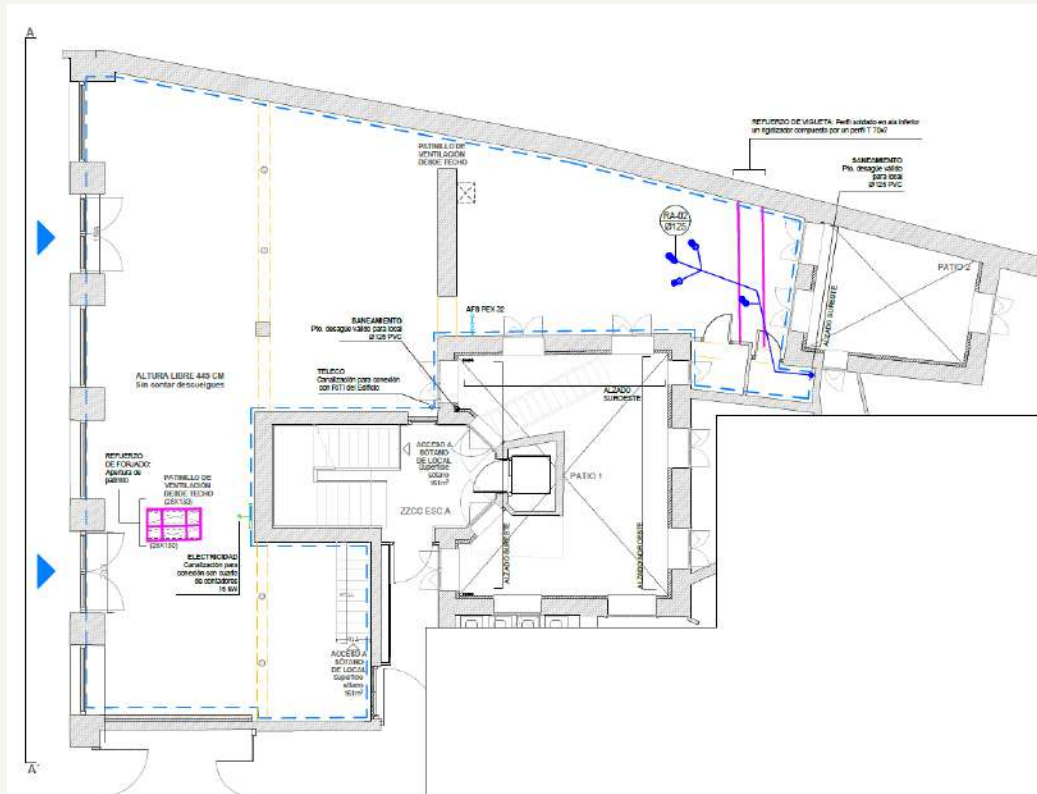
Planta Calle 176,21 m 2
