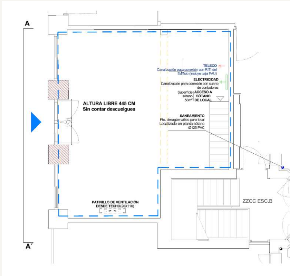
Planta Calle 56,48 m 2
